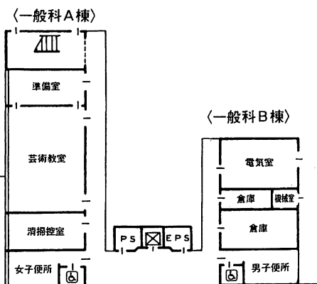
《1階平面図》
