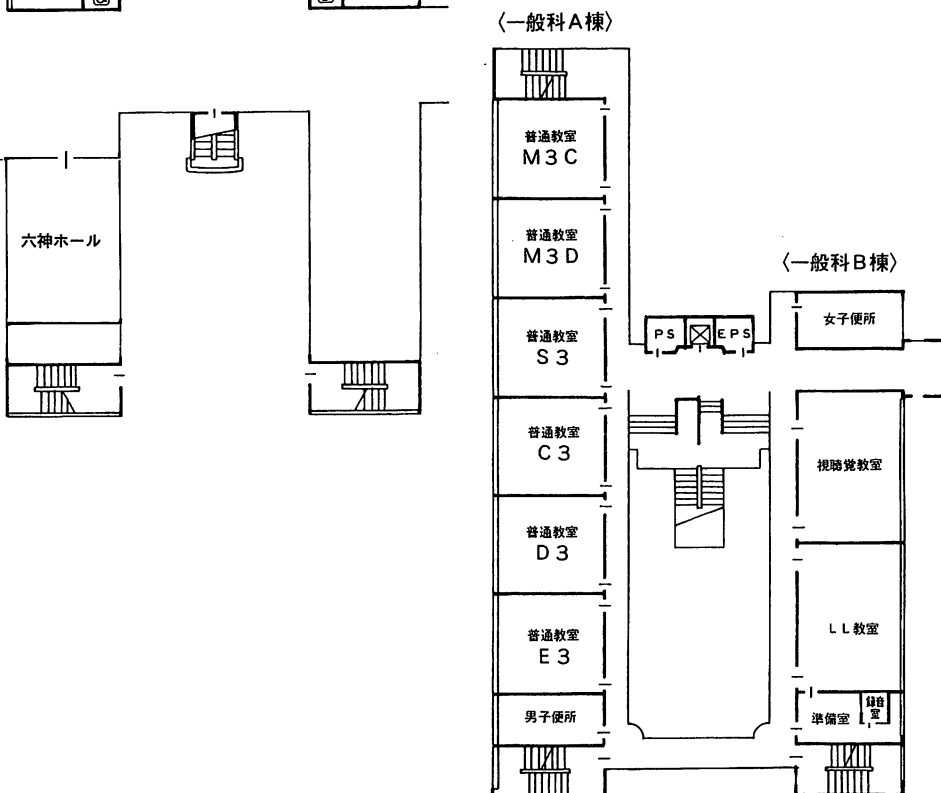
《2階平面図》
