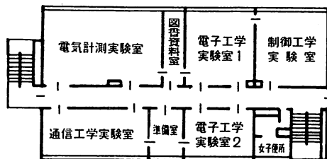
《2階平面図》
