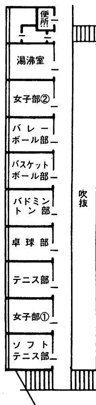
《 2 階平面図 》
