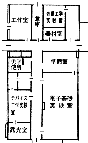
《1 階平面図》
