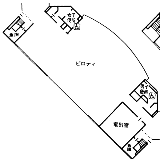
《1階平面図》
